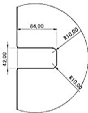
CAM KESİM DETAYI
